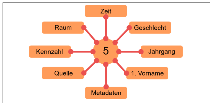
Abbildung 12: Datenpunkte beschreiben
