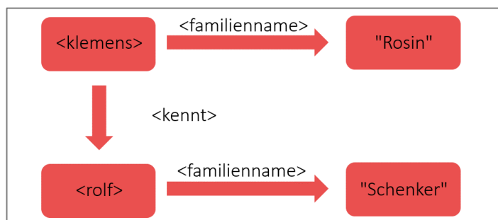
Abbildung 3: Graph
