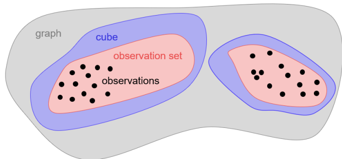
Abbildung 13: Datenstrukturen
