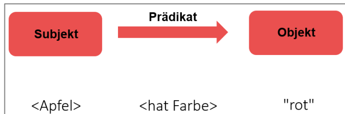
Abbildung 2: Triple
